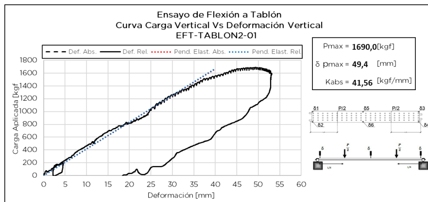
Figura 7.1.6 Respuesta de ensayos de Probeta EFT-TABLON2-01
