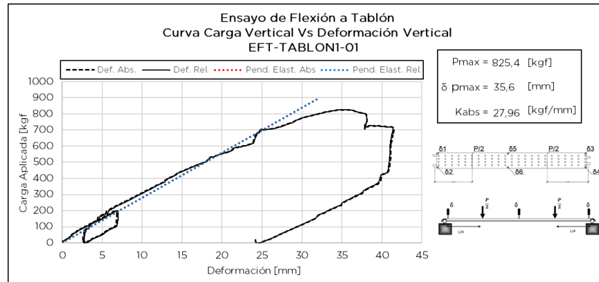
Figura 7.1.4 Respuesta de ensayos de Probeta EFT-TABLON1-01
