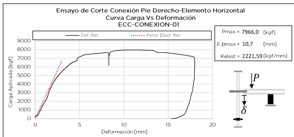
Figura 7.14.3 Respuesta de ensayo ECC-CONEXIÓN-01
