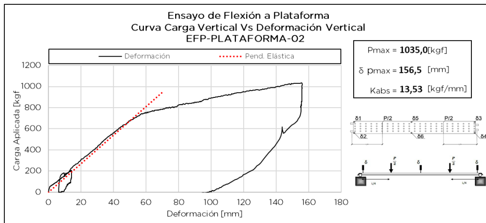
Figura 7.2.3 Respuesta de ensayos de Probeta EFP-PLATAFORMA-02
