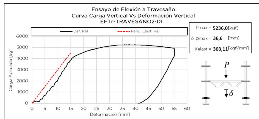
Figura 7.3.6 Respuesta de ensayo EFTr-TRAVESAÑO2-01
