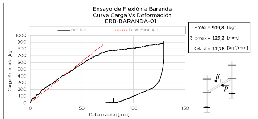
Figura 7.6.3 Respuesta de ensayos ERB-BARANDA-01
