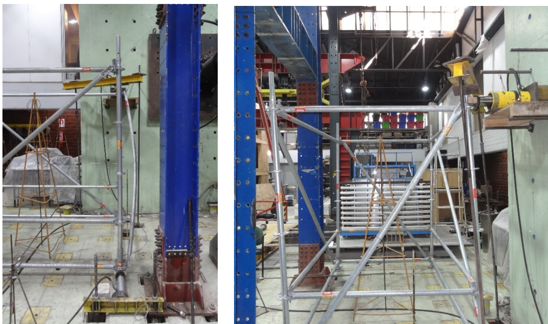
Figura 7.8.6 Estado final Probeta EAT-ARRIOSTRAMIENTO-02
