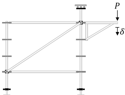
Figura 7.18.1 Esquema ensayo
