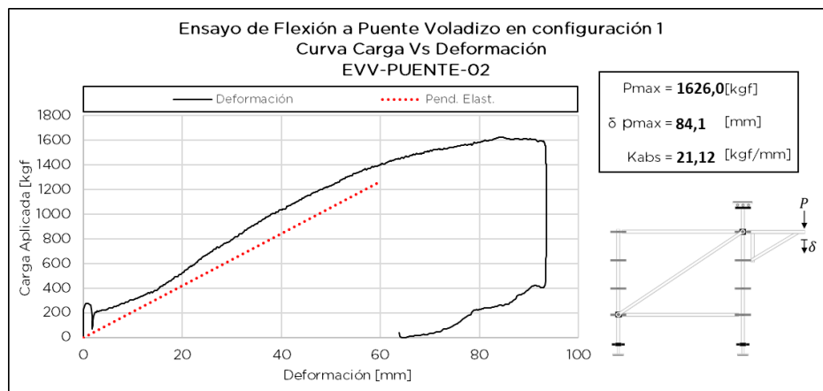
Figura 7.18.5 Respuesta de ensayo EVV-PUENTE-02
