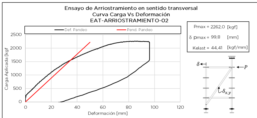
Figura 7.8.5 Respuesta de ensayo EAT-ARRIOSTRAMIENTO-02
