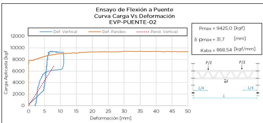
Figura 7.17.5 Respuesta de ensayo EVP-PUENTE-02
