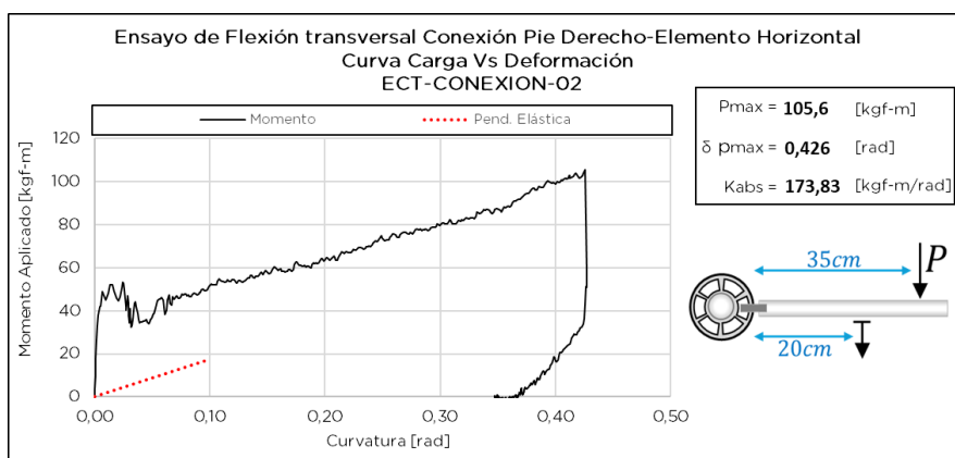
Figura 7.16.4 Respuesta de ensayo EFT-CONEXIÓN-02
