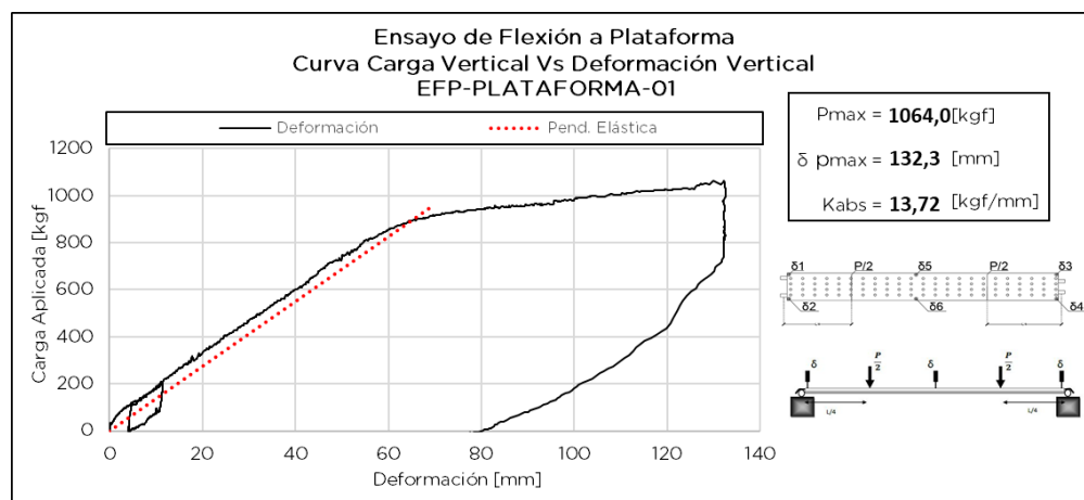
Figura 7.2.2 Respuesta de ensayos de Probeta EFP-PLATAFORMA-01
