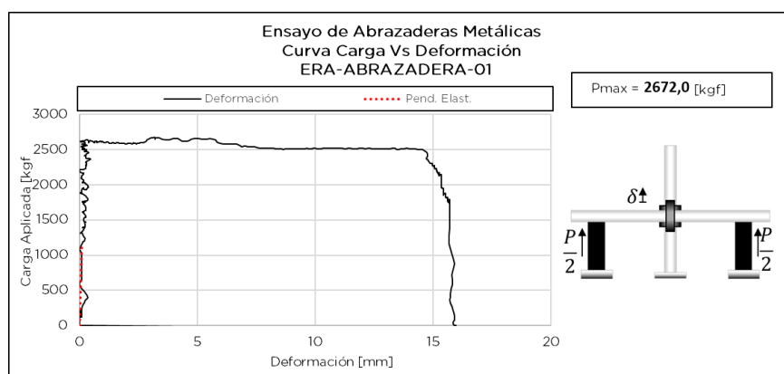
Figura 7.19.4 Respuesta de ensayo ERA-ABRAZADERA-01
