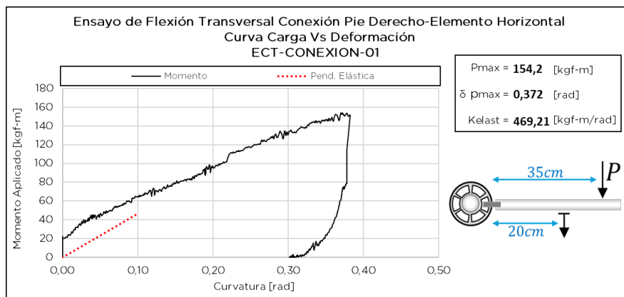
Figura 7.16.3 Respuesta de ensayo EFT-CONEXIÓN-01
