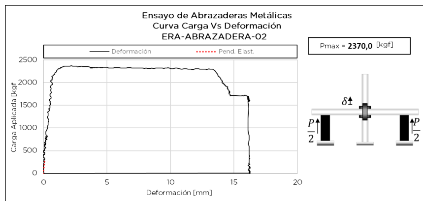
Figura 7.19.5 Respuesta de ensayo ERA-ABRAZADERA-02
