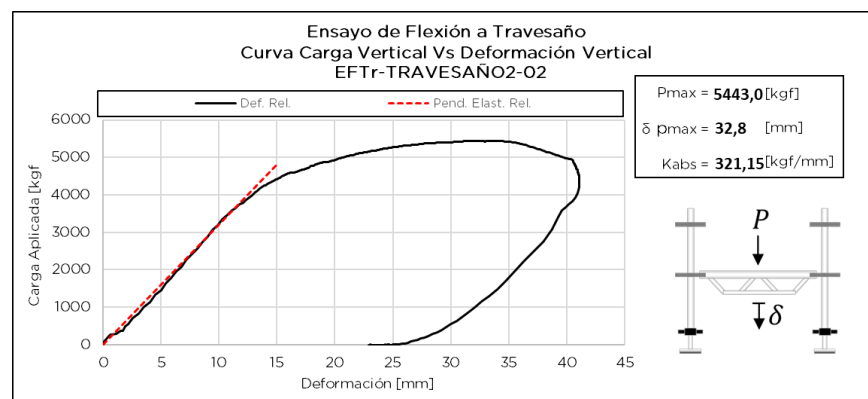
Figura 7.3.7 Respuesta de ensayo EFTr-TRAVESAÑO2-02
