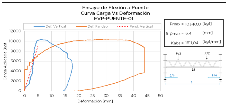
Figura 7.17.4 Respuesta de ensayo EVP-PUENTE-01
