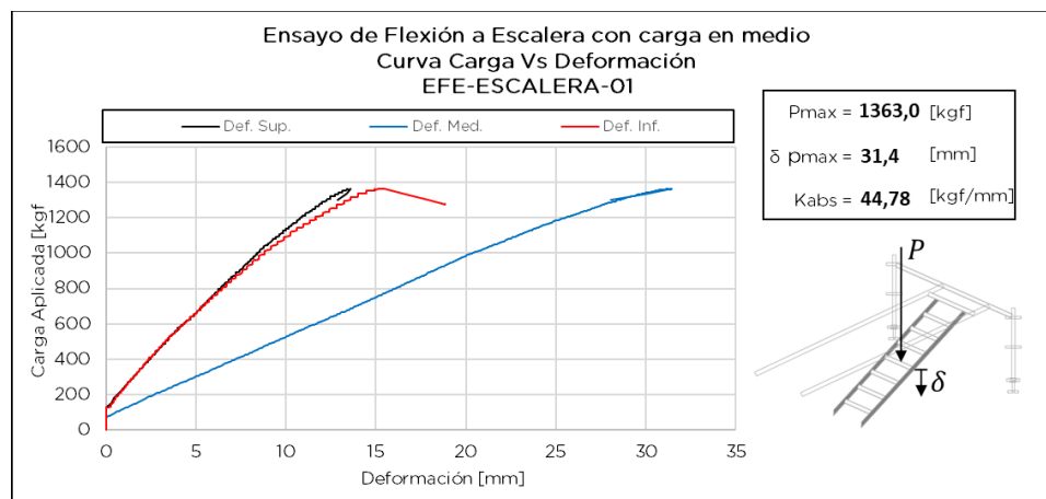
Figura 7.10.4 Respuesta de ensayo EFE-ESCALERA-01
