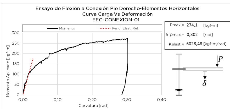
Figura 7.15.3 Respuesta de ensayo EFC-CONEXIÓN-01
