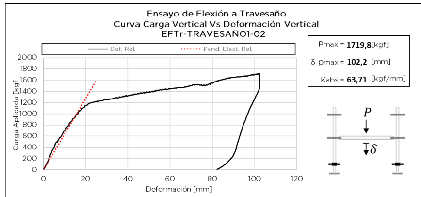
Figura 7.3.5 Respuesta de ensayo EFTr-TRAVESAÑO1-02
