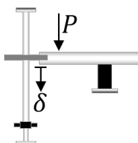
Figura 7.14.1 Esquema ensayo
