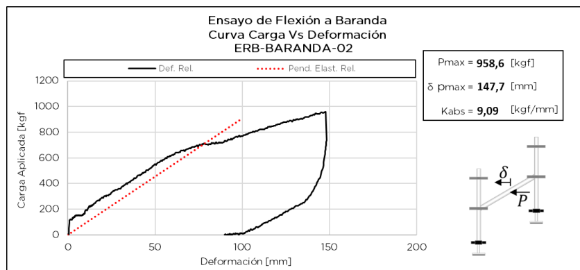
Figura 7.6.4 Respuesta de ensayos ERB-BARANDA-02
