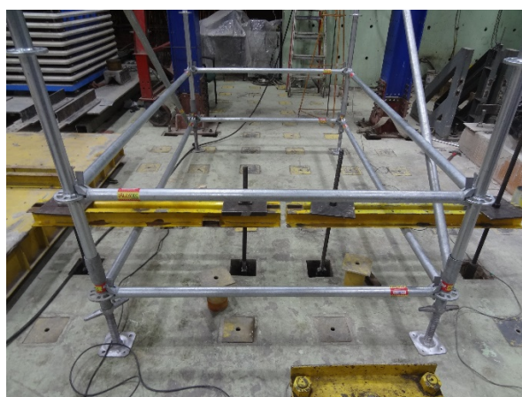
Figura 7.18.3 Anclaje para evitar levantamiento
