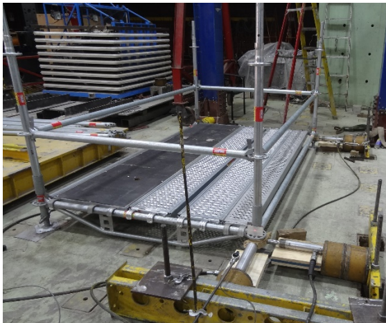
Figura 7.13.2 Montaje del ensayo
