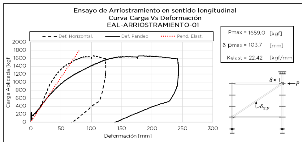
Figura 7.7.4 Respuesta de ensayo EAL-ARRIOSTRAMIENTO-01
