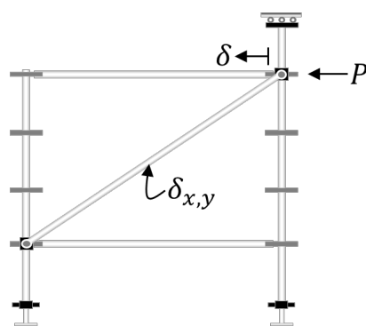
Figura 7.7.1 Esquema ensayo
