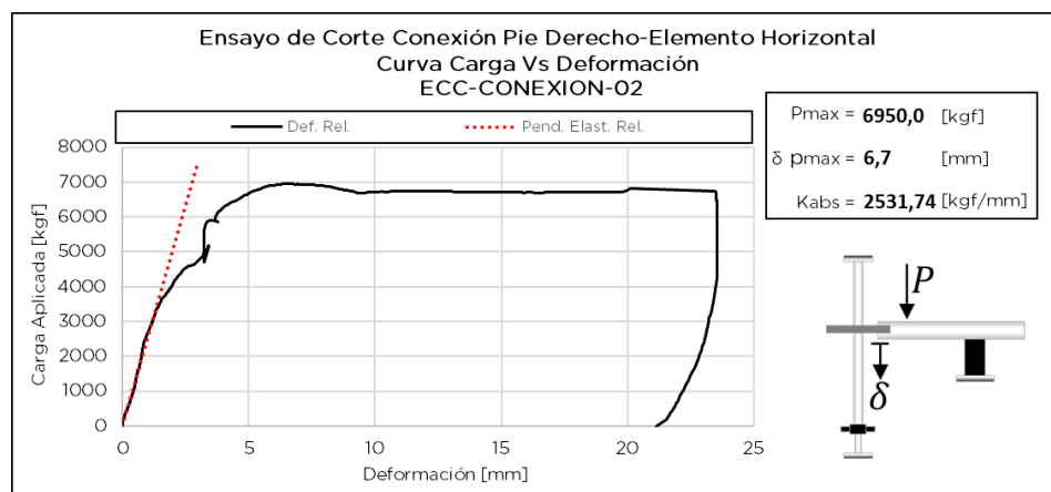
Figura 7.14.4 Respuesta de ensayo ECC-CONEXIÓN-02
