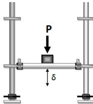
Figura 7.3.1 Esquema ensayo
