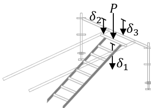
Figura 7.12.1 Esquema ensayo
