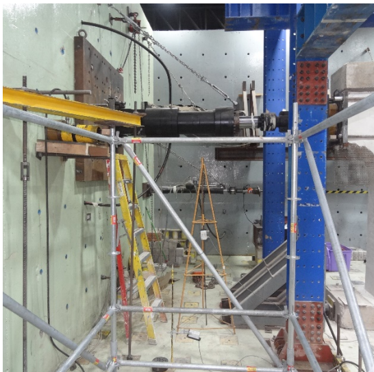
Figura 7.8.2 Montaje del ensayo
