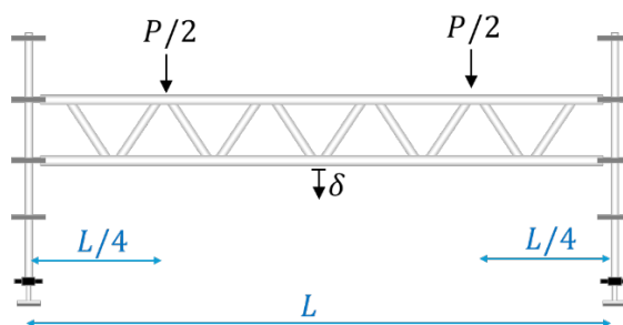
Figura 7.17.1 Esquema ensayo
