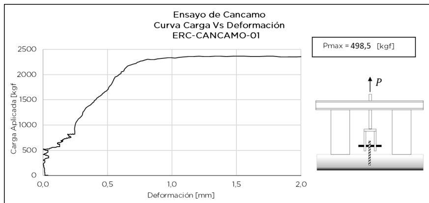
Figura 7.20.4 Respuesta de ensayo ERC-CANCAMO-01
