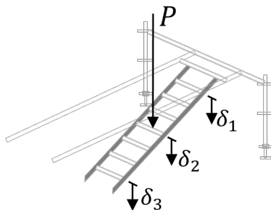
Figura 7.10.1 Esquema ensayo
