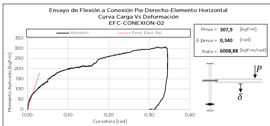
Figura 7.15.4 Respuesta de ensayo EFC-CONEXIÓN-02
