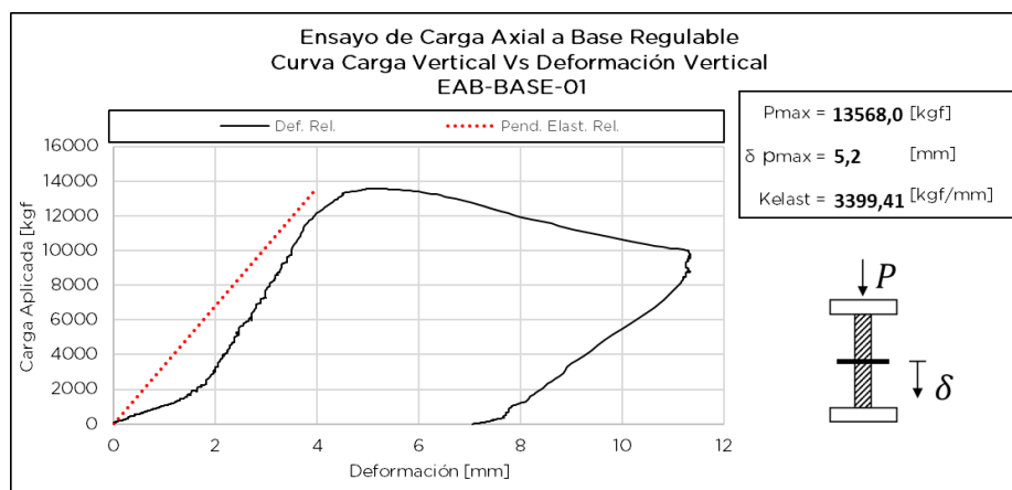
Figura 7.5.3 Respuesta de ensayos Probeta EAB-BASE-01
