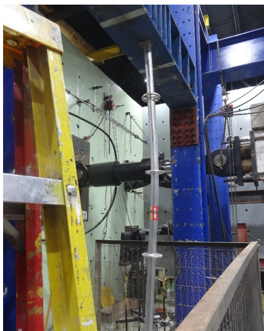
Figura 7.4.6 Estado final Probeta ECP-PIEDERECHO-01
