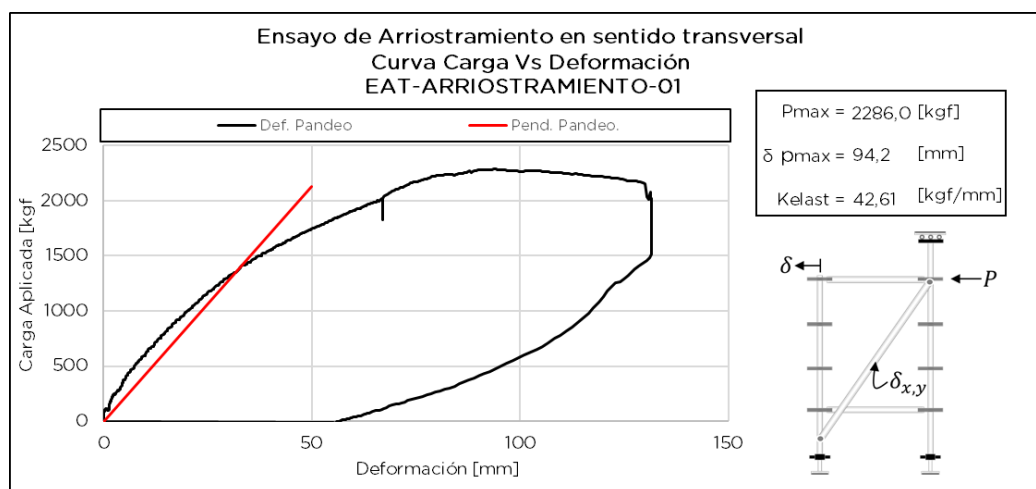
Figura 7.8.4 Respuesta de ensayo EAT-ARRIOSTRAMIENTO-01
