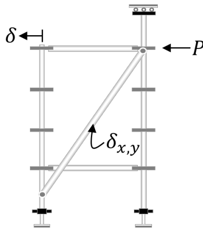
Figura 7.8.1 Esquema ensayo
