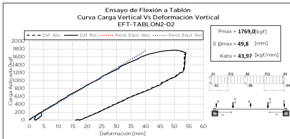
Figura 7.1.7 Respuesta de ensayos de Probeta EFT-TABLON2-02
