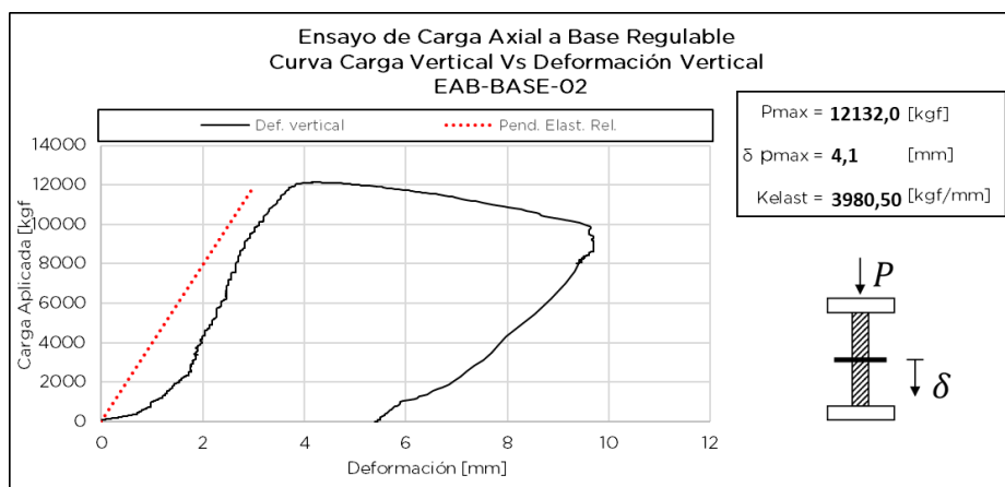
Figura 7.5.4 Respuesta de ensayos Probeta EAB-BASE-02
