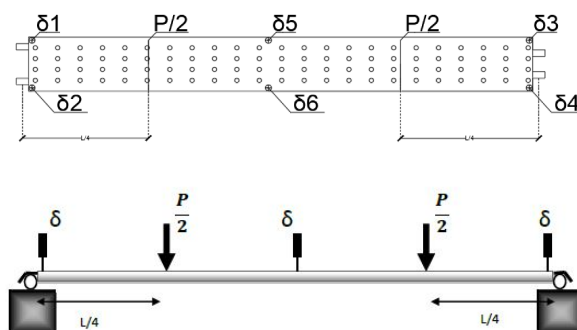
Figura 7.1.1 Esquema ensayo
