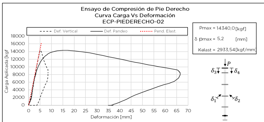
Figura 7.4.5 Respuesta de ensayo Probeta ECP-PIEDERECHO-02
