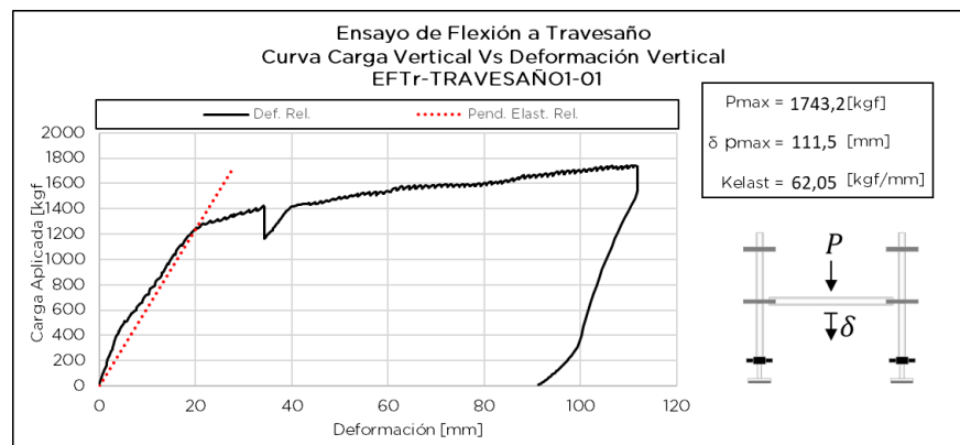
Figura 7.3.4 Respuesta de ensayo EFTr-TRAVESAÑO1-01
