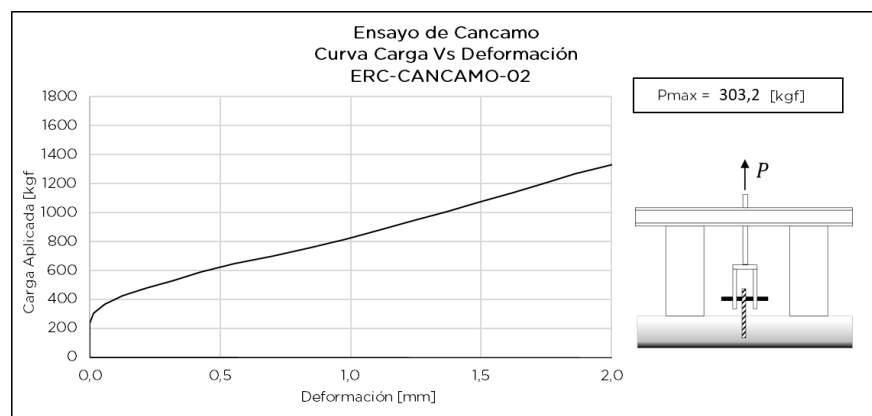
Figura 7.20.5 Respuesta de ensayo ERC-CANCAMO-02
