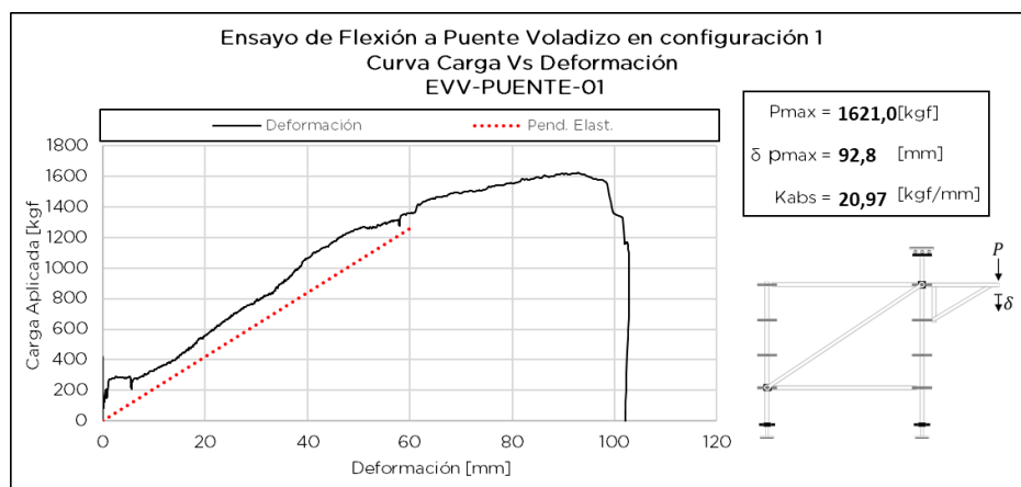
Figura 7.18.4 Respuesta de ensayo EVV-PUENTE-01
