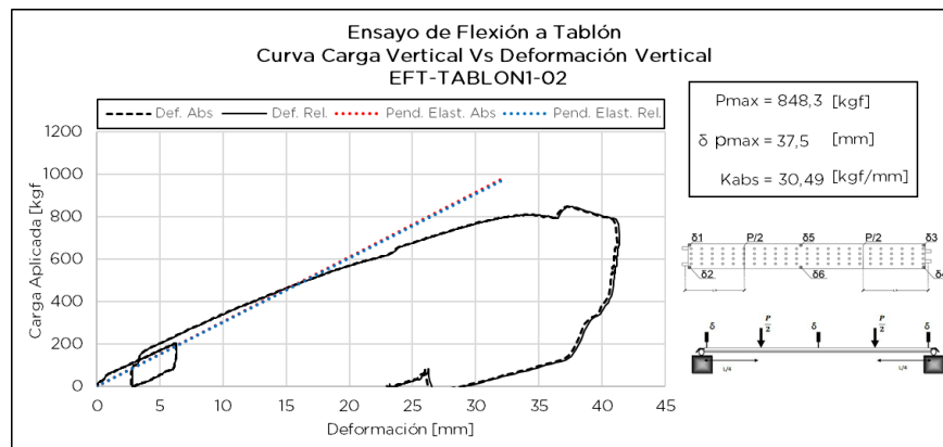
Figura 7.1.5 Respuesta de ensayos de Probeta EFT-TABLON1-02
