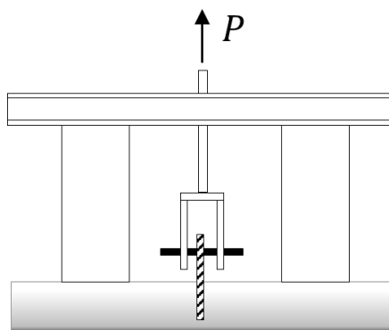
Figura 7.20.1 Esquema ensayo
