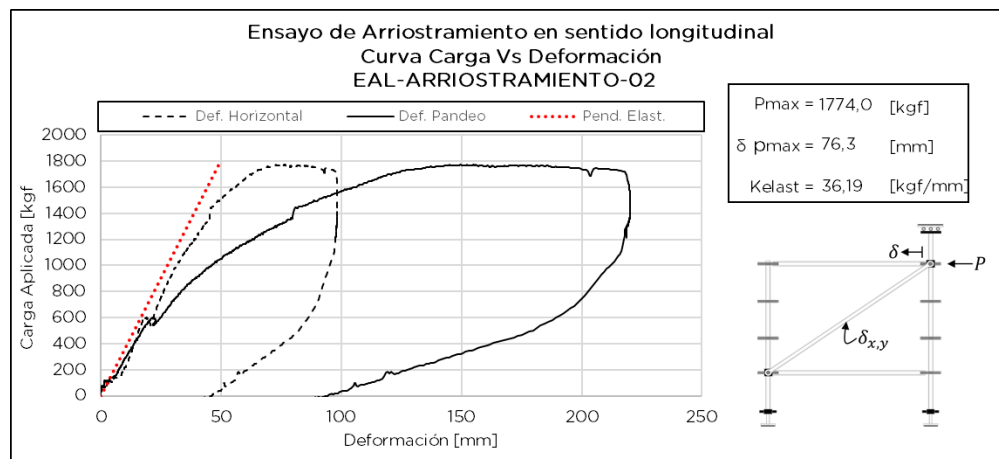
Figura 7.7.5 Respuesta de ensayo EAL-ARRIOSTRAMIENTO-02
