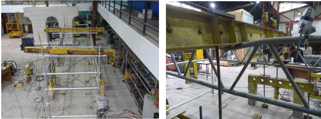
Figura 7.17.6 Estado final probeta EVP-PUENTE-01
