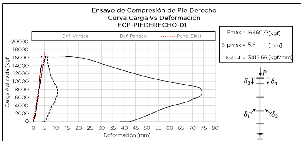
Figura 7.4.4 Respuesta de ensayo Probeta ECP-PIEDERECHO-01
